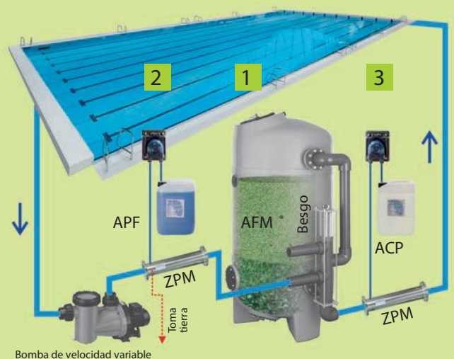
Circuito filtración DAISY para piscinas públicas.
